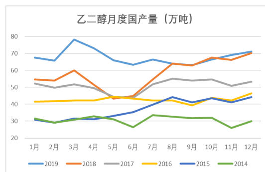
图 4. 乙二醇产量
