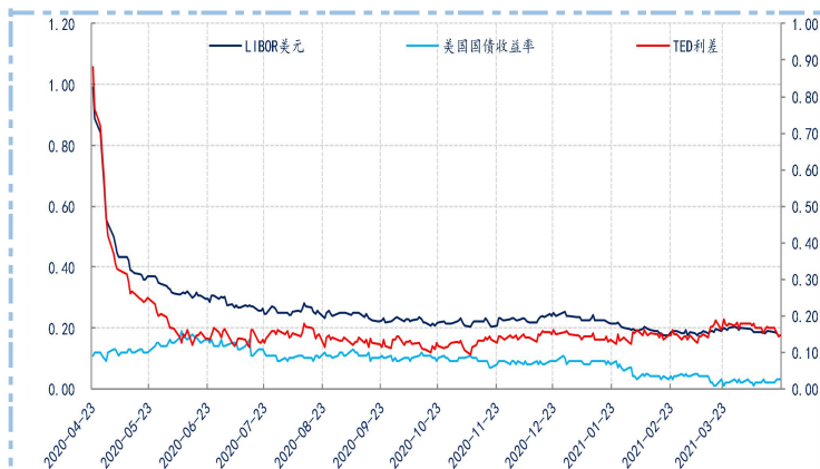
图 3. TED 利差
