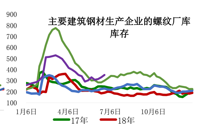
图 24: 螺纹厂库
