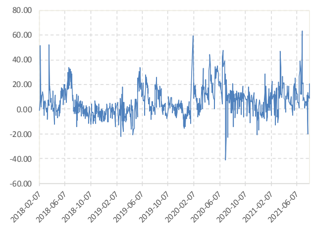
图 12: IH 主力合约基差 单位: 点
