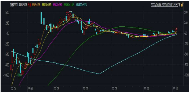
图 3：郑棉 301-郑棉 305
