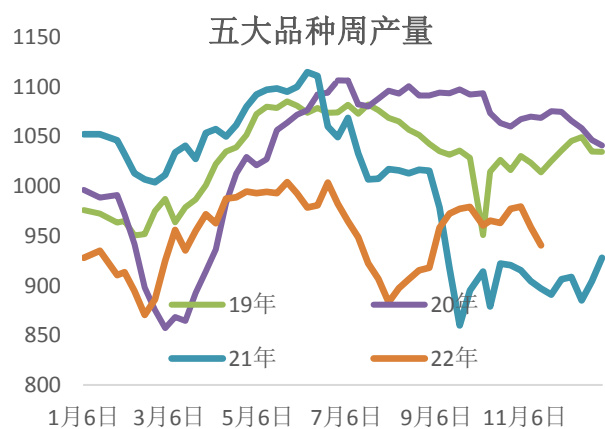
图 6: 五大钢材周度产量 单位: 万吨
