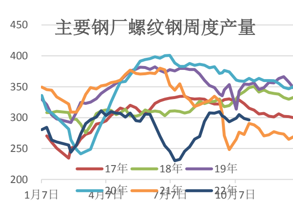
图 5: 主要钢厂螺纹钢周度产量 单位: 万吨
