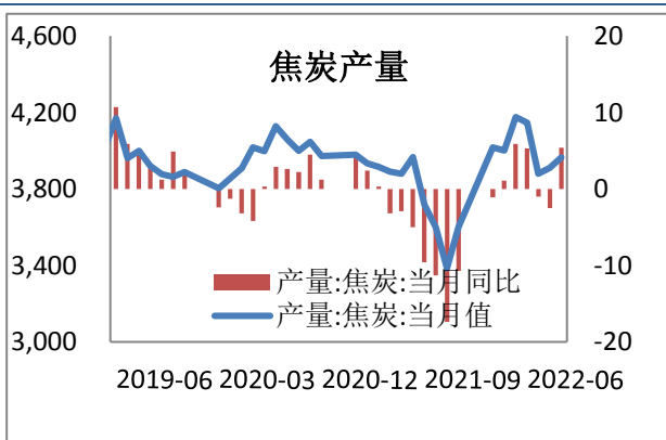
图 13: 焦炭产量走势图 单位: 万吨
