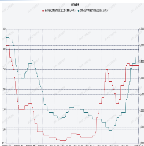
图 1 锌矿加工费
