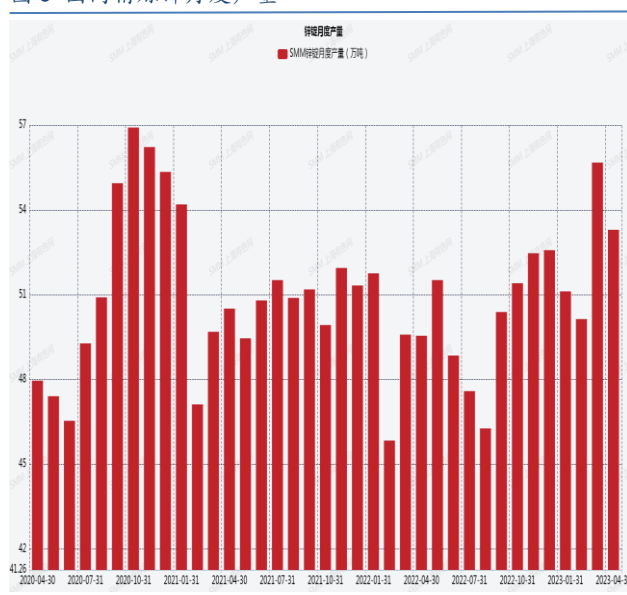
图 5 国内精炼锌月度产量
