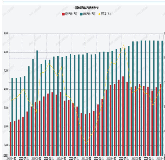
图 8 中国电解铝建成产能与运行产能
