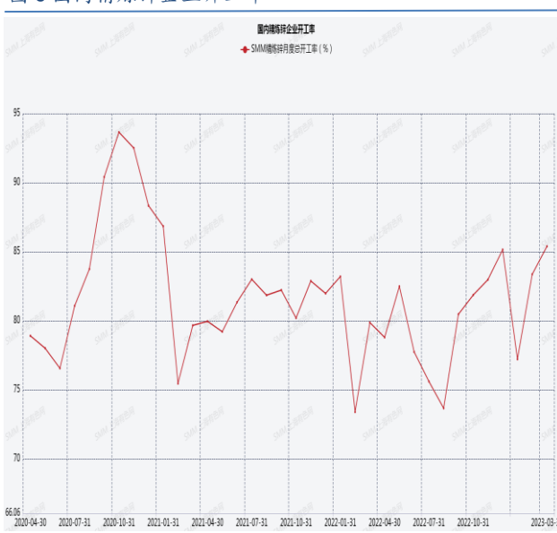
图 6 国内精炼锌企业开工率
