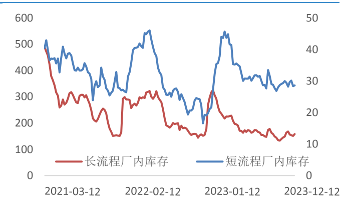
图 35: 长短流程厂内库存 单位: 万吨
