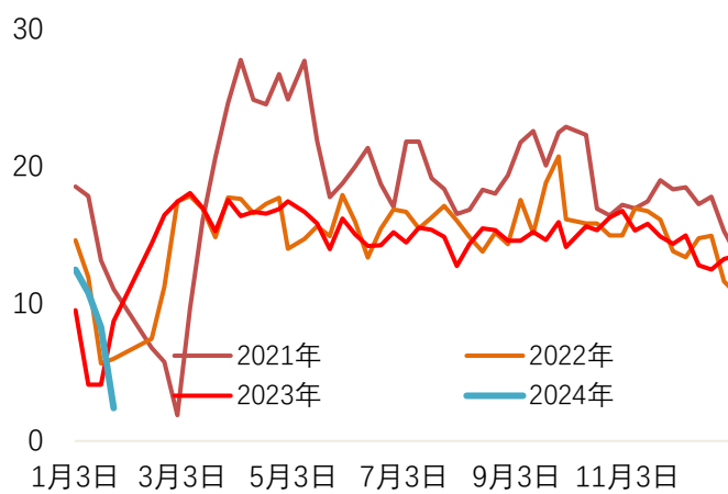
图 24: 唐山钢厂高炉检修影响产量
