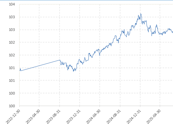
图 11: 2 年期国债期货连续合约 单位: 元
