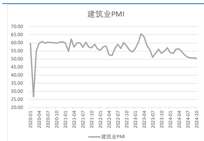
图 37: 建筑业PMI
